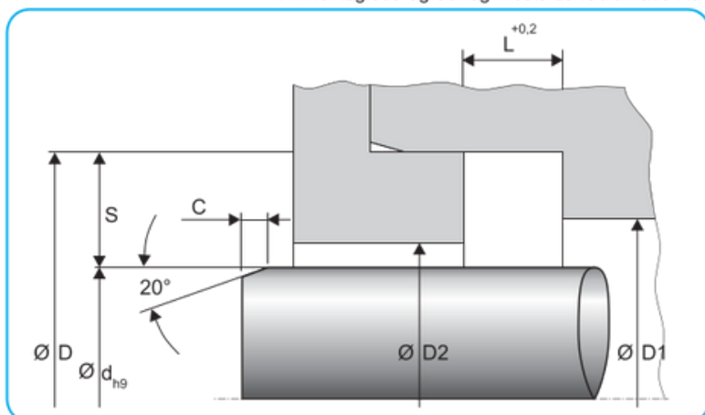
Primer izgleda ugradnog mesta za radimatic R35
